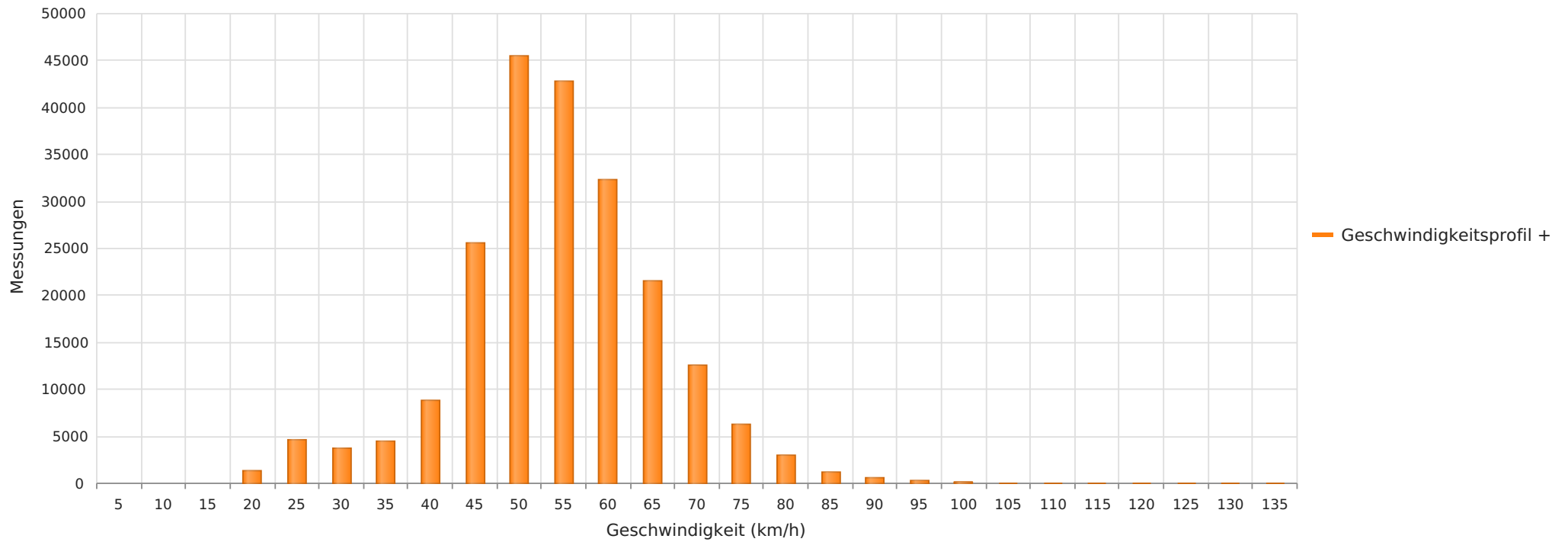
2023_08_29-09_29 Essel K105 Richtung Ortskern Anzahl der Messwerte vs. Geschwindigkeit
