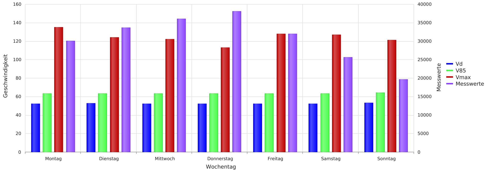
2023_08_29-09_29 Essel K105 Richtung Ortskern Vd, V85, Vmax, Anzahl der Messwerte vs. Wochentag
