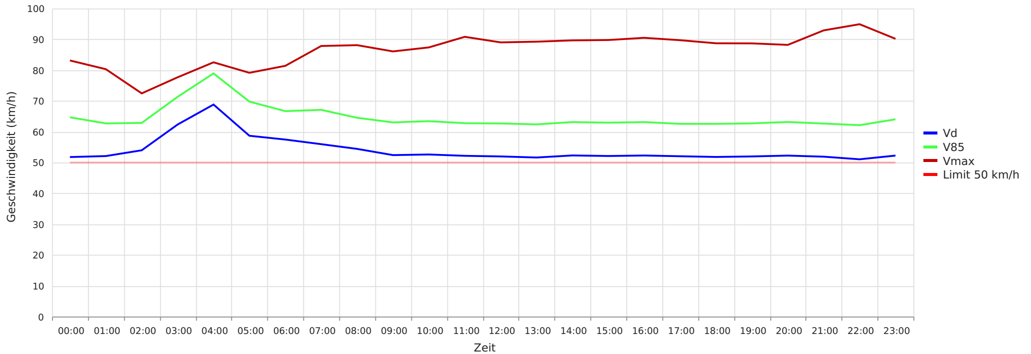
2023_08_29-09_29 Essel K105 Richtung Ortskern Vd, V85, Vmax vs. Uhrzeit
