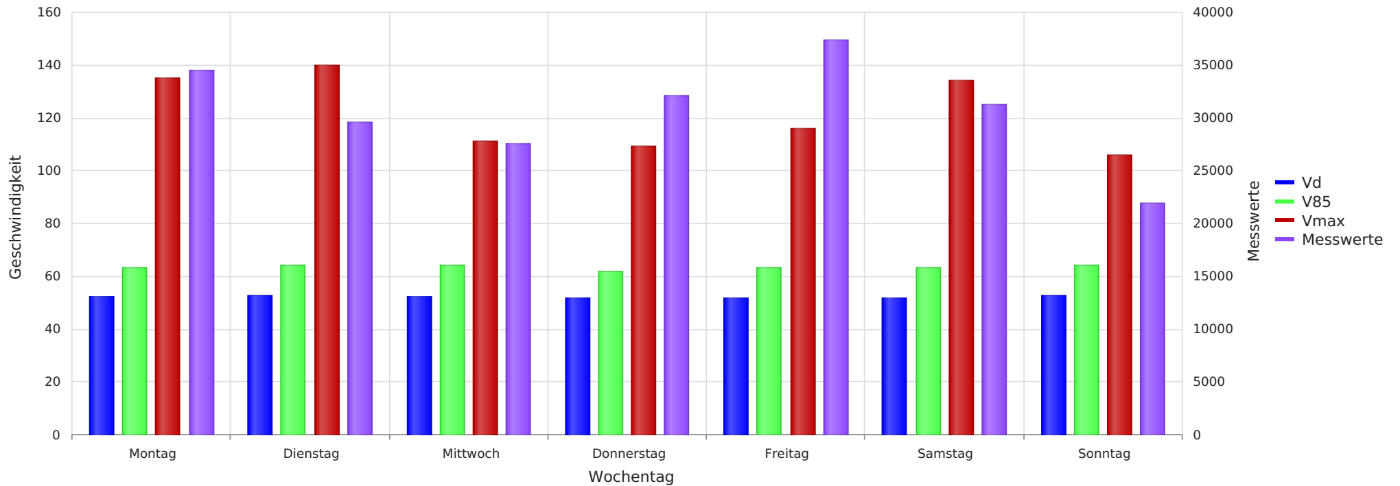
2023_07_27-08_29 Essel K105 Richtung Ortskern Vd, V85, Vmax, Anzahl der Messwerte vs. Wochentag
