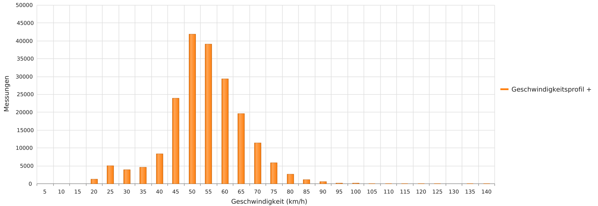
2023_07_27-08_29 Essel K105 Richtung Ortskern Anzahl der Messwerte vs. Geschwindigkeit
