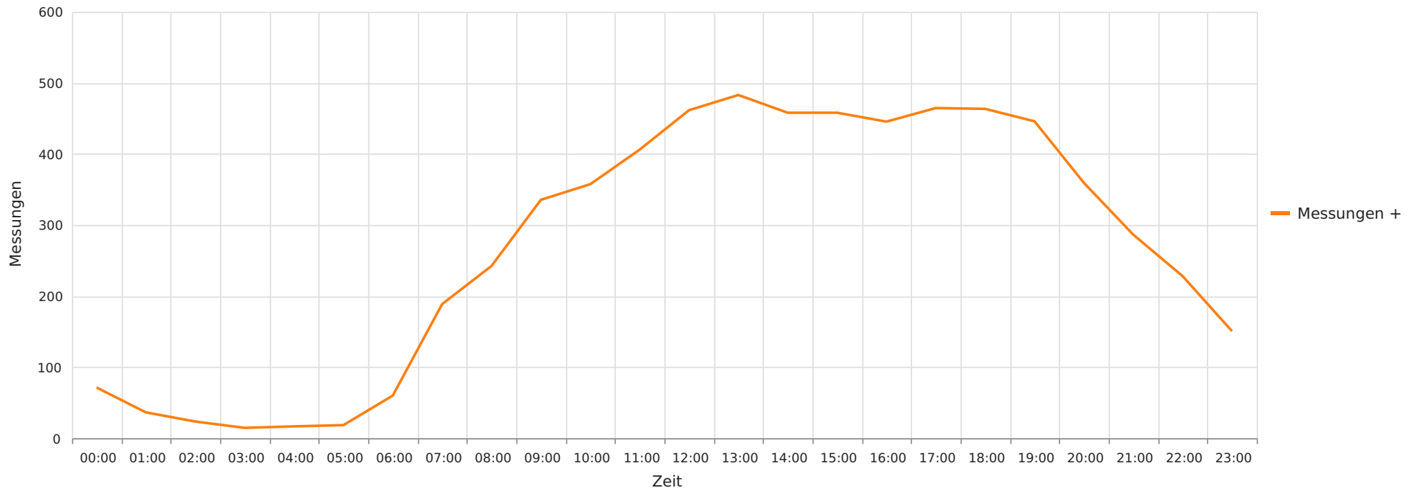
2023_07_27-08_29 Essel K105 Richtung Ortskern Gemittelte Anzahl an Messwerten vs. Uhrzeit
