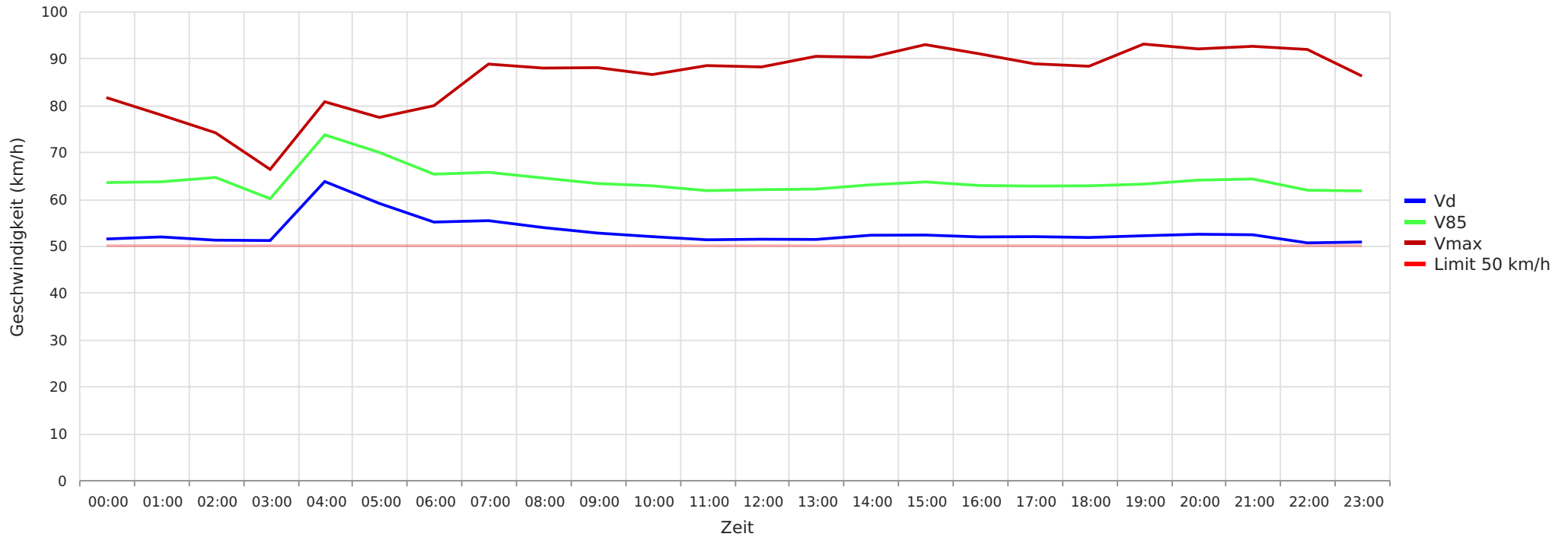
2023_07_27-08_29 Essel K105 Richtung Ortskern Vd, V85, Vmax vs. Uhrzeit
